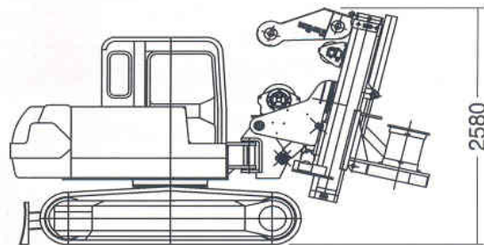
Dimensioni per il trasporto / Dimensions for transport Dimensions pour le transport / Dimensiones para el transporte
